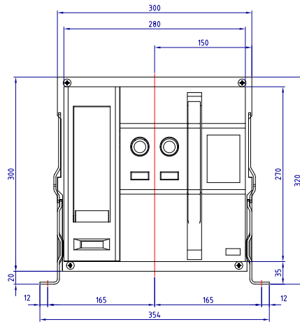
AN 630/1600 3P Fixed ACB
